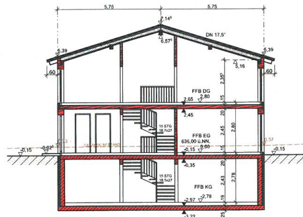
SCHNITT A-A
