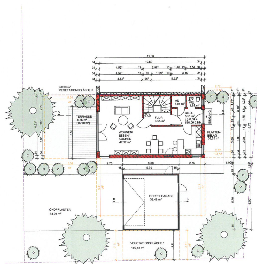
ERDGESCHOSS
