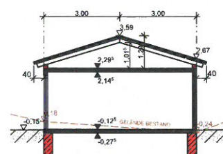
SCHNITT B-B
