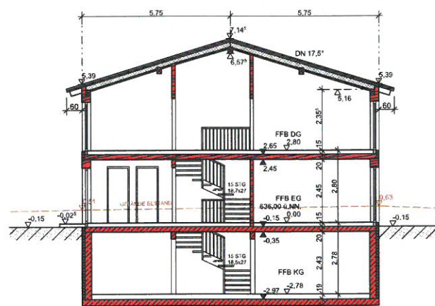
SCHNITT A-A
