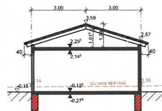
SCHNITT B-B
