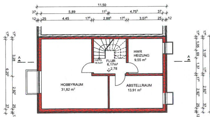
KELLERGESCHOSS
