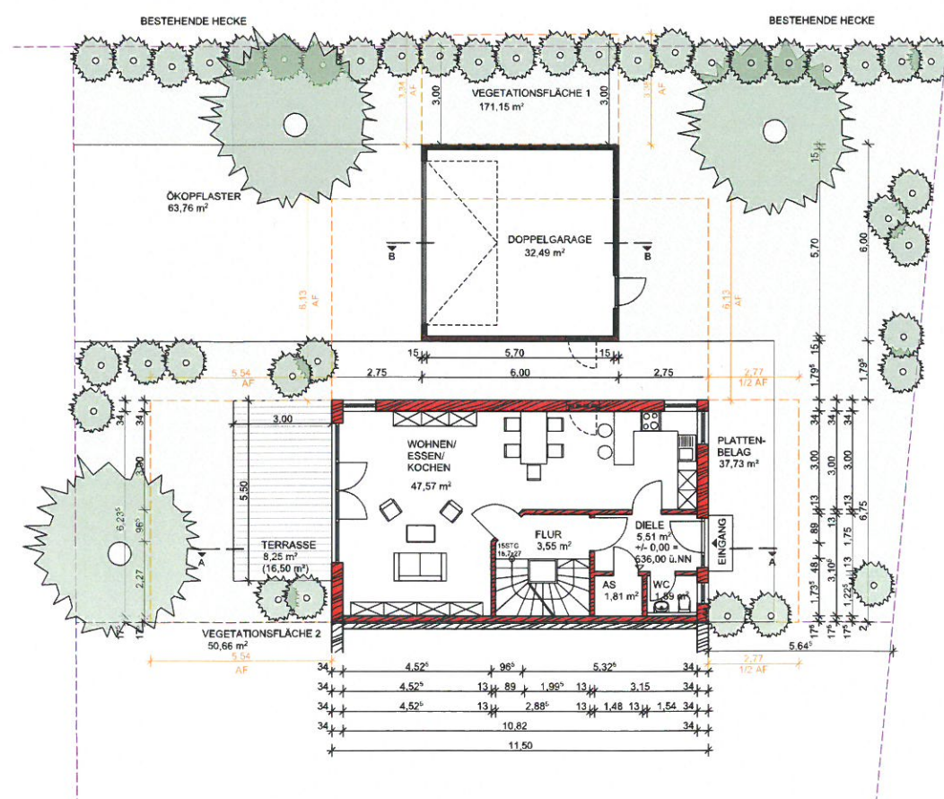
ERDGESCHOSS
