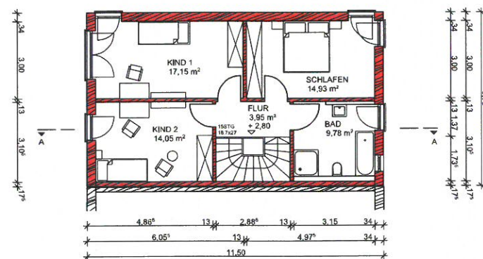
DACHGESCHOSS
