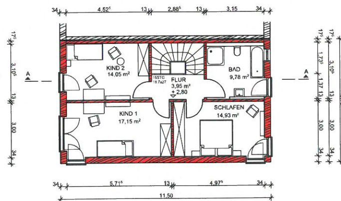
DACHGESCHOSS
