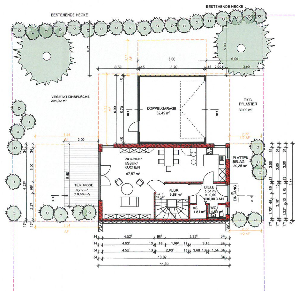
ERDGESCHOSS
