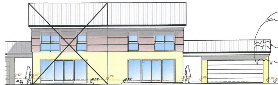
ANSICHT WEST
