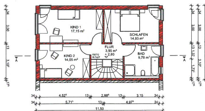
DACHGESCHOSS
