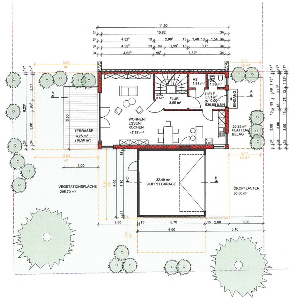
ERDGESCHOSS
