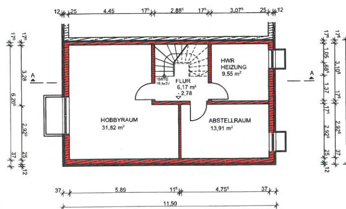
KELLERGESCHOSS
