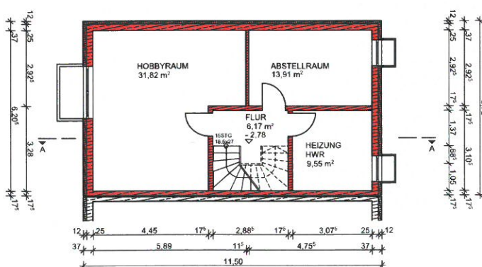
KELLERGESCHOSS
