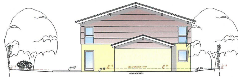
ANSICHT SÜD
