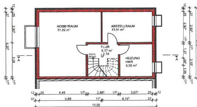
KELLERGESCHOSS
