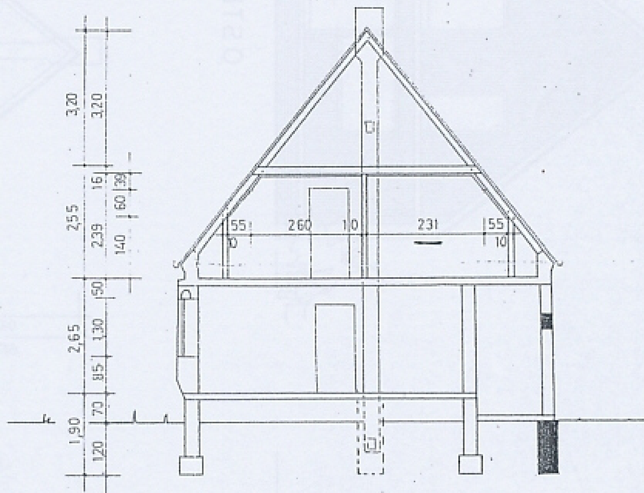
SCHNITT A-A
